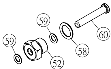
52-60 頂針銅罩組 2 AS451-52-60
