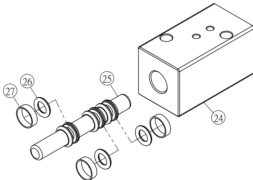
24-27 方型轉換閥組 1 AS451-24-27
