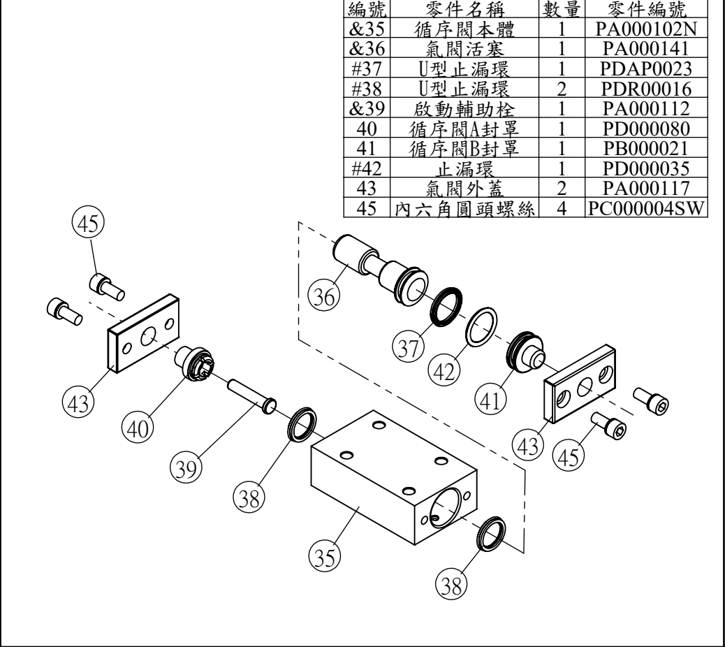
35-45 循序閥組 1 DS03-35-45
